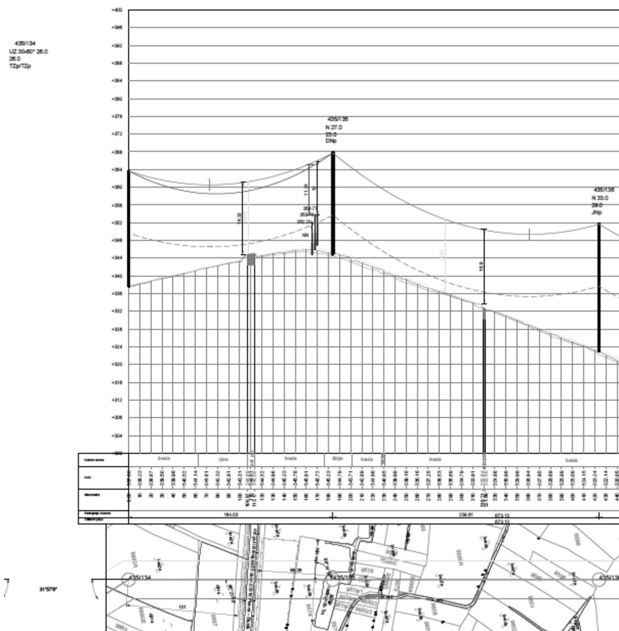
Профил трасе предметног ДВ у распону 435/134 - 435/135 (локација 9).
