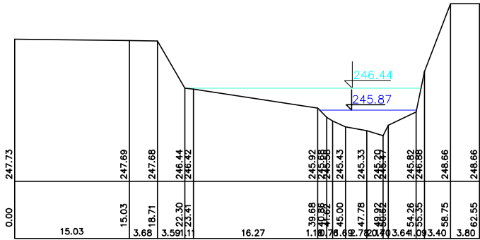
Prof.br. 2 Stacionaža 0+099.60 R=1:100/500
