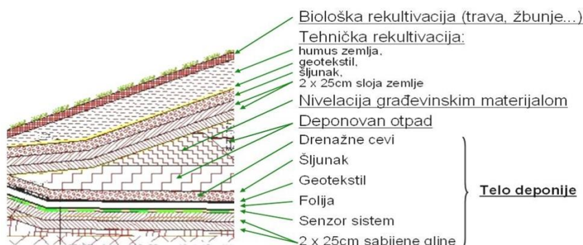
Слика бр.1: Пресек слојева тела депоније
