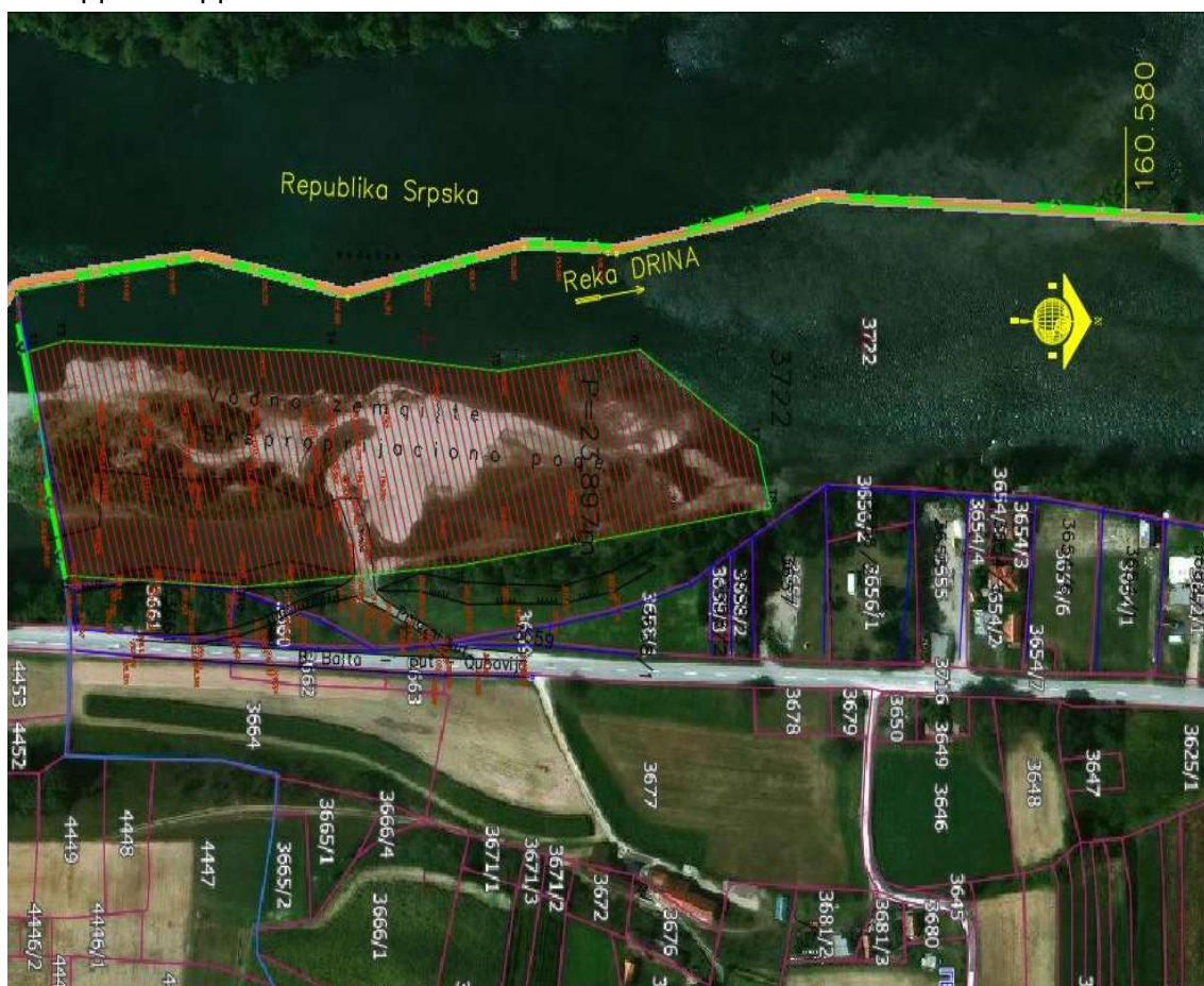
Орто-фото снимак ( http://www.geosrbija.rs/ ) експлоатационог поља на стационажи од км160+580 го км 161+085
